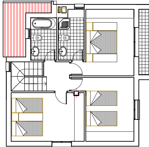
PLANTA PRIMERA
